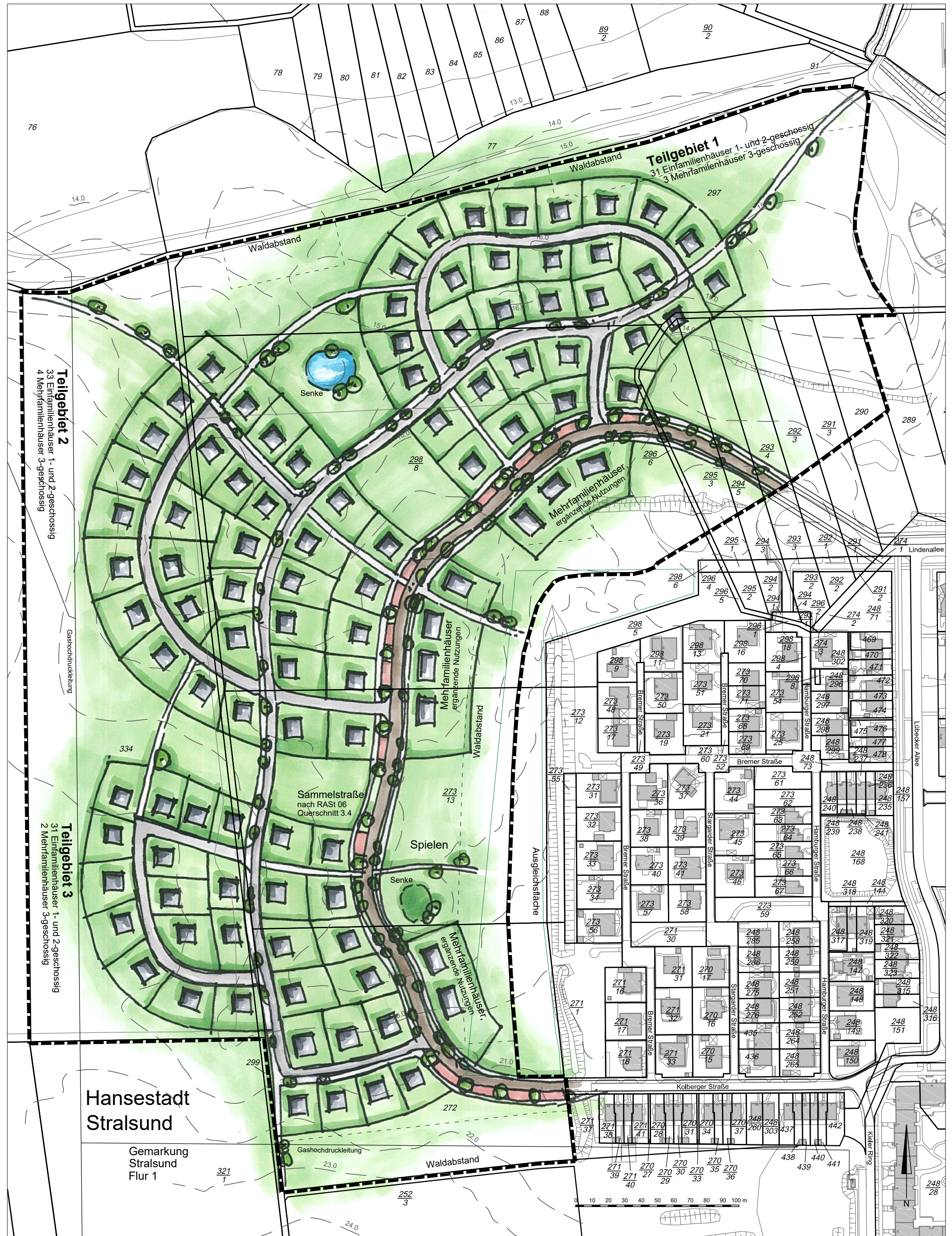
Bebauungsplan Nr. 39 „Wohngebiet westlich der Lindenallee, Freienlande“ der Hansestadt Stralsund Städtebauliches Konzept - Variante 5a Maßstab 1:2000 bei A3 Datum: Juni 2017
